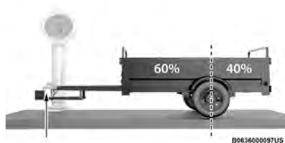
Distribución del peso
