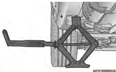
Posición frontal de elevación con gato
