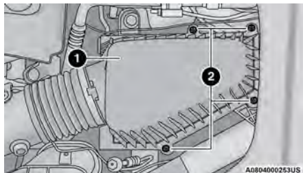
Cubierta, filtro de aire del motor
