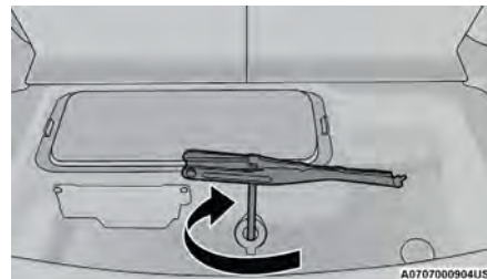
Rotación de la llave del cabrestante
