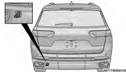
Anilla para remolque trasera instalada
