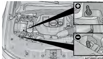
Bornes para el arranque con puente
