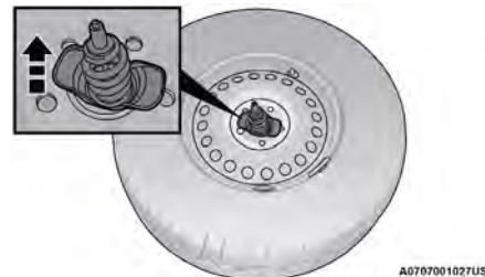
Instalación del cabrestante
