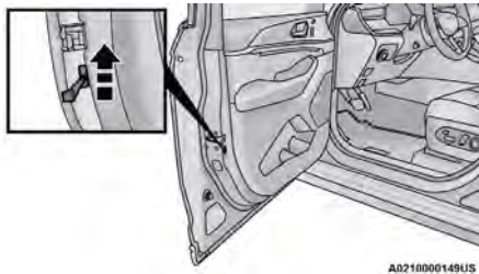
Palanca de bloqueo de emergencia (se muestra la puerta del conductor)
