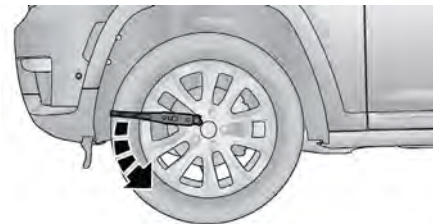
Afloje las tuercas de la rueda
