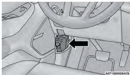
Ubicación de la correa de liberación manual de la posición de estacionamiento
