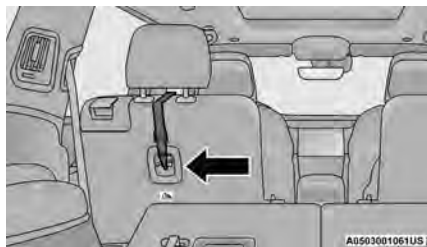
Montaje de la correa de atadura superior del asiento tipo capitán (asiento para 6 pasajeros)
