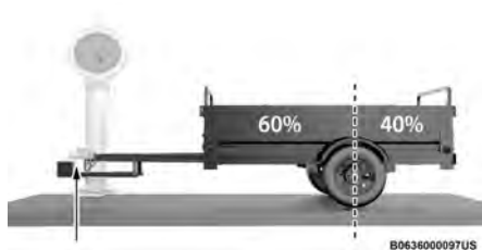
Distribución del peso
