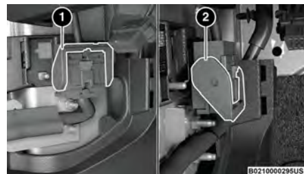
Mazo de cables de la puerta delantera
