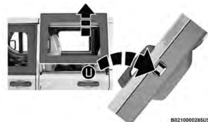
Retire la semipuerta superior y limpie la parte inferior del hueco de la puerta.
