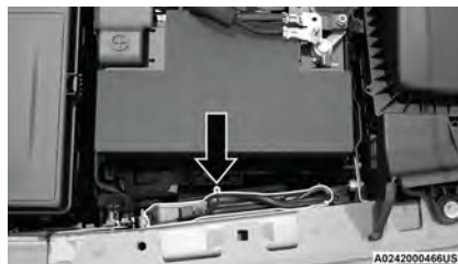
Conexiones del interruptor auxiliar - Debajo del capó
