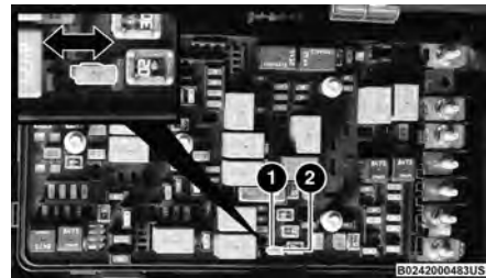
Ubicación de los fusibles de las tomas de corriente
